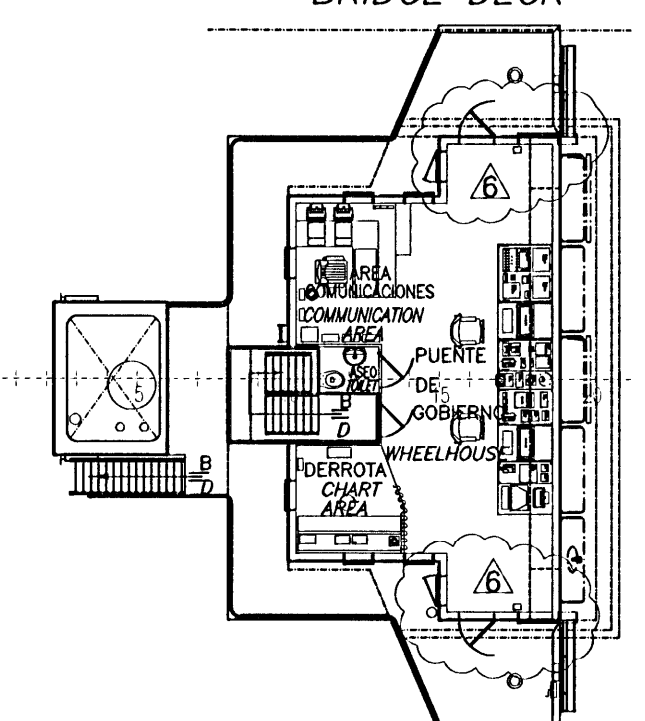
CUBIERTA PUENTE BRIDGE DECK
