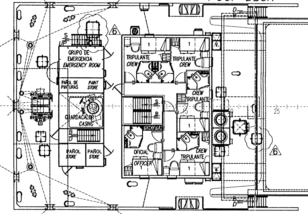
CUBIERTA TOLDILLA POOP DECK
