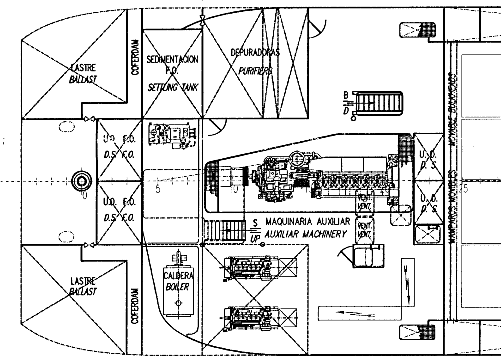
PLATAFORMA DE MAQUINAS ENGINE PLATFORM
