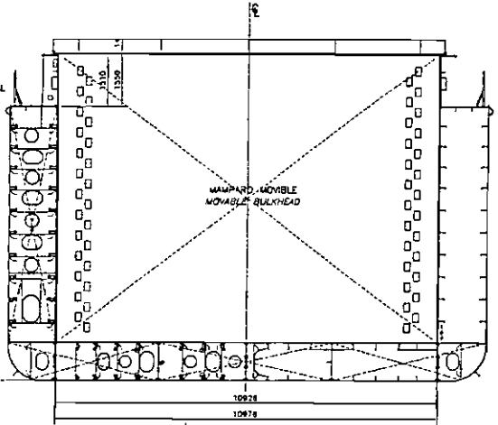
SECCION POR MAMPARO MOVIBLE MOVABLE BULKHEAD SECTION
