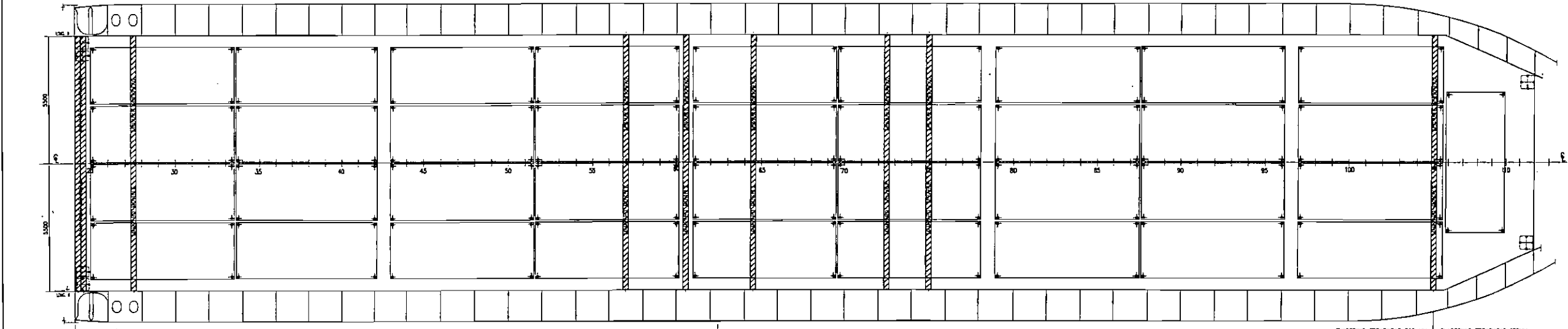
DOBLE FONDO DOUBLE BOTTOM
